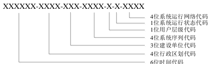
图2 系统代码结构图
